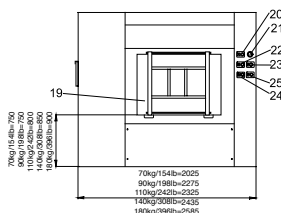
ВИД СЗАДИ МВ 70 90 110 140 180
