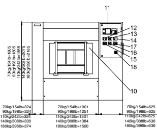
ВИД СЗАДИ МВ 70 90 110 140 180
