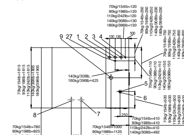
ВИД СБОКУ МВ 70 90 110 140 180
